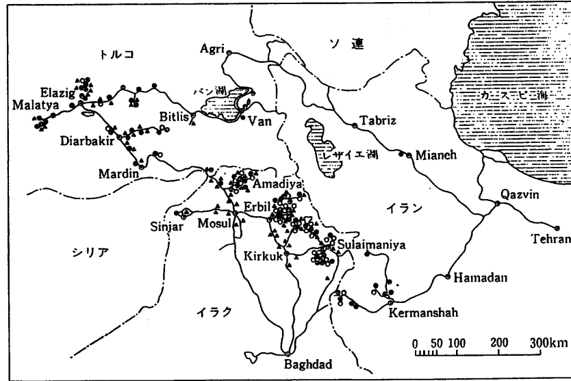
図2 イラク・トルコおよびイランにおける野生四倍性コムギ (○)、 野生一粒系コムギ (●)およびクサビコムギ (▲) の採集地点
